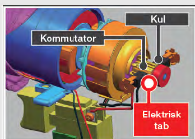
KONVENTIONEL MOTOR
